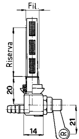
Figura 9 M 10x1 Conico 1:6
