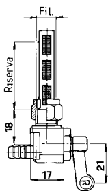
Figura 10 M 10x1 Conico 1:6
