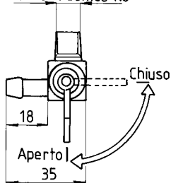
Figura 9 M 10x1 Conico 1:6
